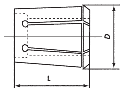
ER Collet
