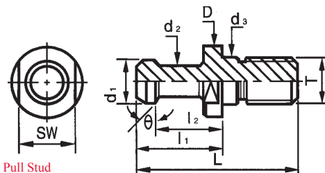
Pull Stud
